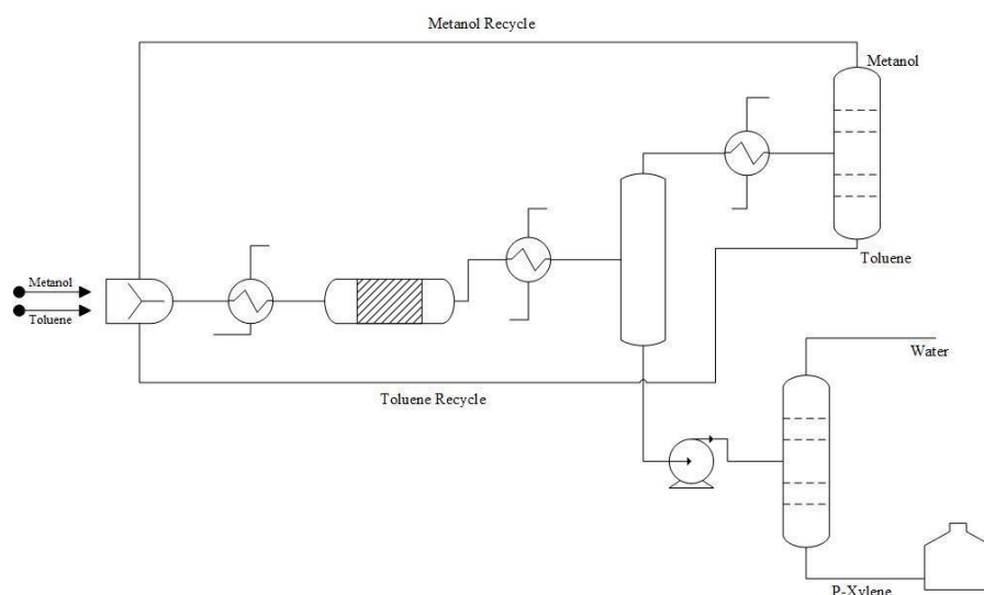
Gambar 1.3 Proses Alkilasi Toluene
