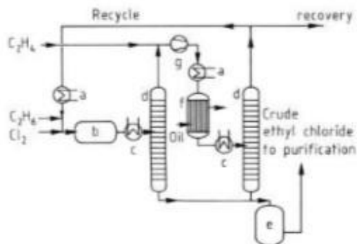
Gambar 1.3 Diagram Alir Proses Klorinasi Etana
