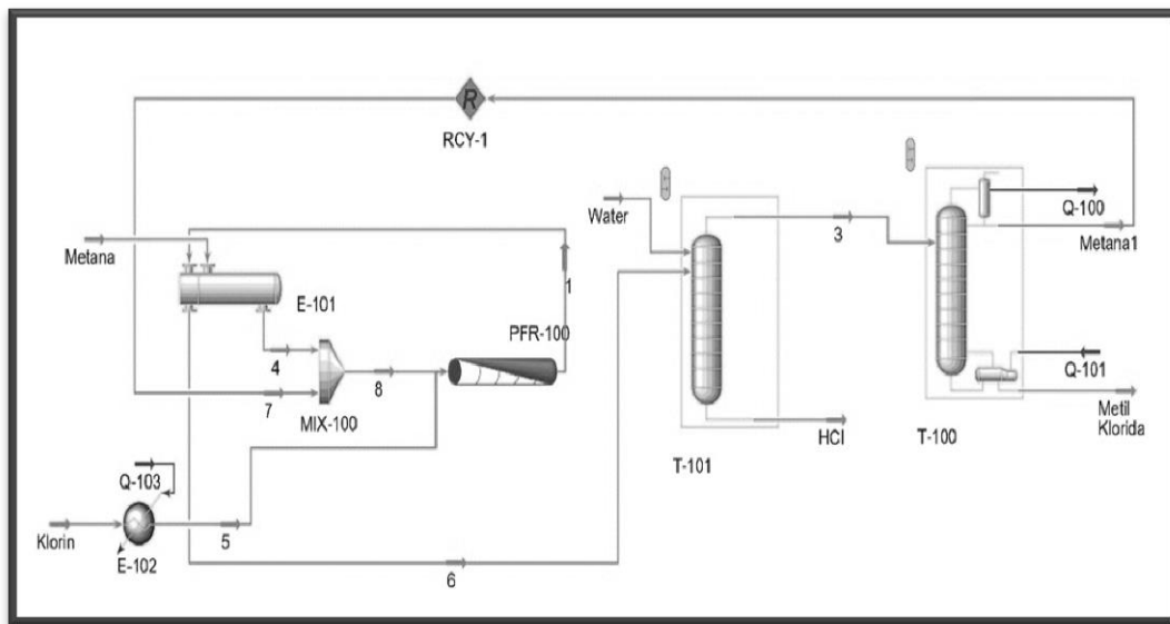
Gambar 1. 3 Flowsheet Metil Klorida dengan Proses Klorinasi Metana Yang Dibuat Ulang Menggunakan Hysys
