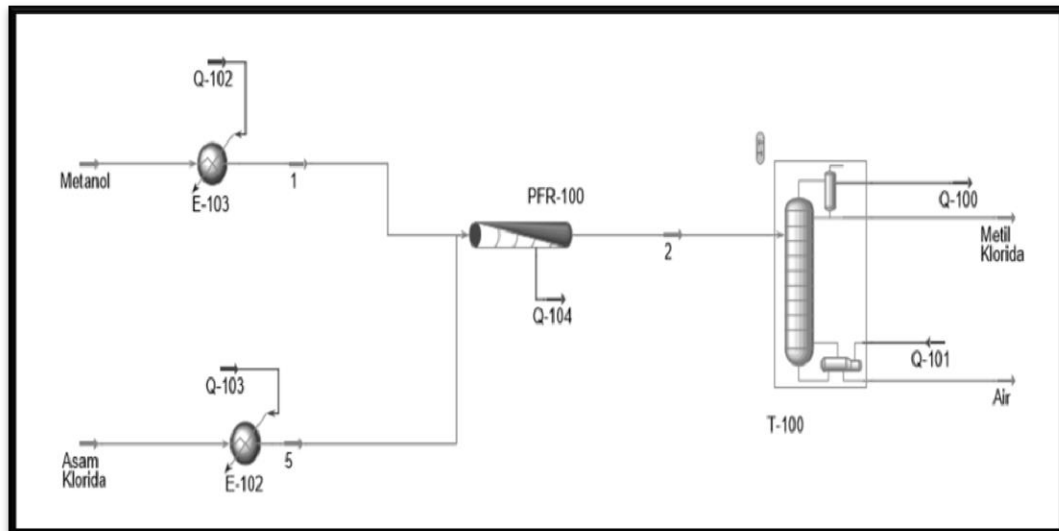
Gambar 1. 2 Flowsheet Metil Klorida Dengan Proses Hidroklorinasi Metanol Yang Dibuat Ulang Menggunakan Hysys
