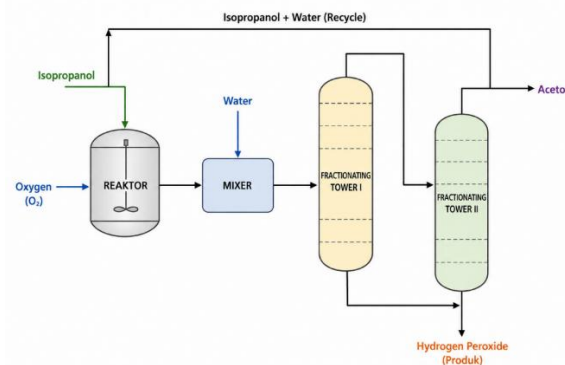
Gambar 1.5 Flowsheet Dasar Proses Esterifikasi (Diadaptasi dari Kirk-Othmer, 2019).
