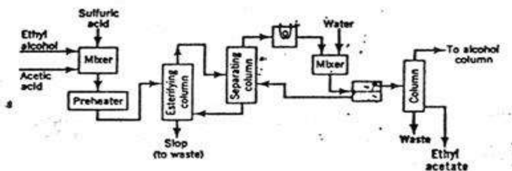
Gambar 1.3 Flowsheet Dasar Proses Esterifikasi
