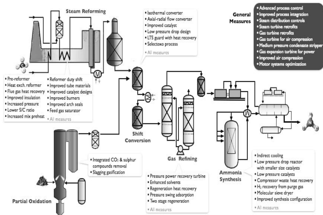
Gambar 1.2 Diagram Alir Dari Proses Haber Bosch Sumber: Mc. Cabe, 1985
