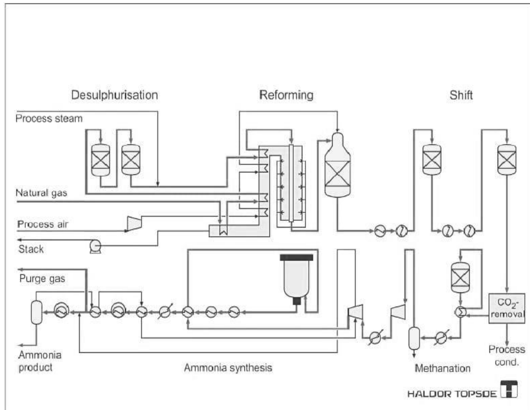
Gambar 1.4 Diagram Alir Dari Proses Haldor-Topsoe Sumber: Mc. Cabe, 1985
